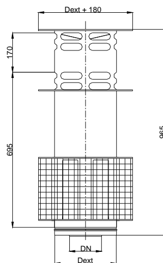
Figure 5 – Terminal concentrique long utilisé avec les versions DINAGAS 3CE+ ou DINAGAS 3CE+ SW.
