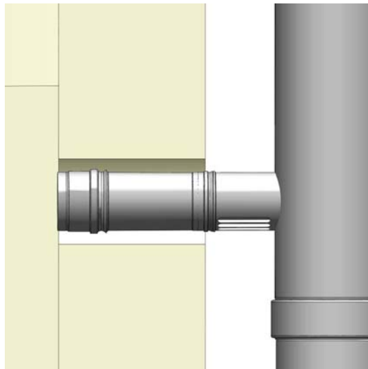
Figure 14 – Conduit de liaison de la version DINAGAS 3CE+ DW (situation extérieure) avec bouchon d'obturation.
