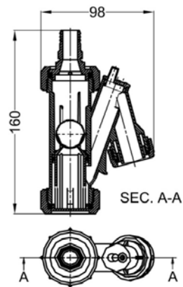
Figure 4 – Collecteur de récupération des condensats du système DINAGAS 3CE+.
