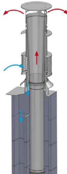
Figure 7 – Pièce d'adaptation du terminal concentrique du système dans sa version DINAGAS 3CE+ SW sur le conduit existant.
