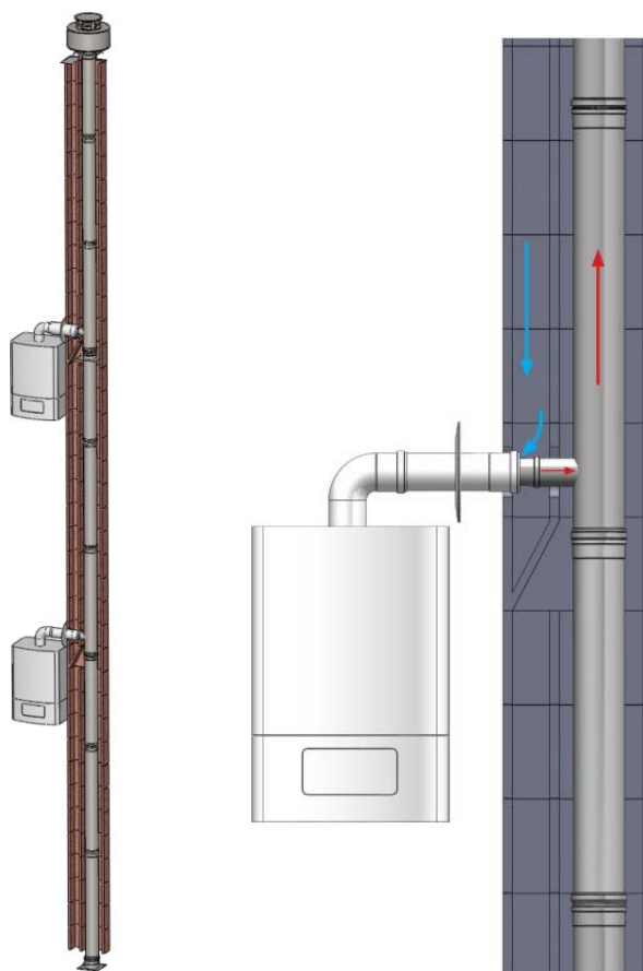
Figure 2 – Principe de montage de la version DINAGAS 3CE+ SW à l'intérieur d'un conduit existant.
