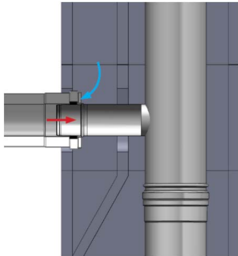
Figure 12 – Mise en place des conduits de liaison, version DINAGAS 3CE+ SW pour rénovation dans un conduit existant.
