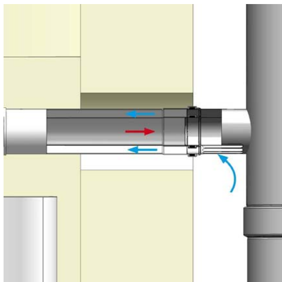
Figure 13 – Mise en place des conduits de liaison, version DINAGAS 3CE+ DW pour utilisation à l'extérieur d'un bâtiment.
