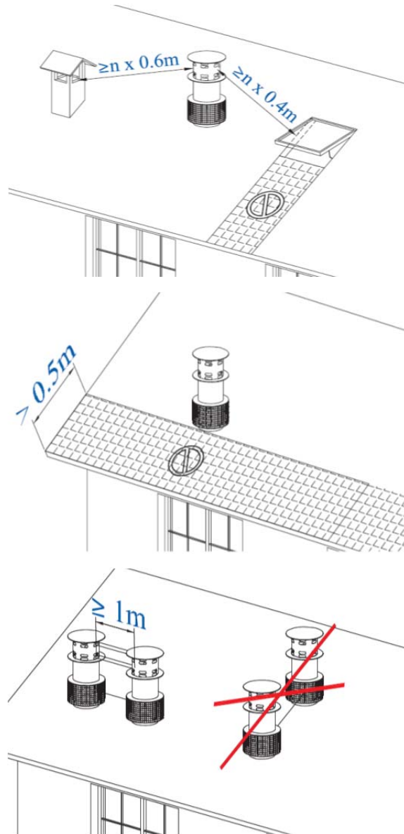
Figure 10 – Positionnement des terminaux en dérogation à l'article 18 de l'arrêté du 22 octobre 1969.
