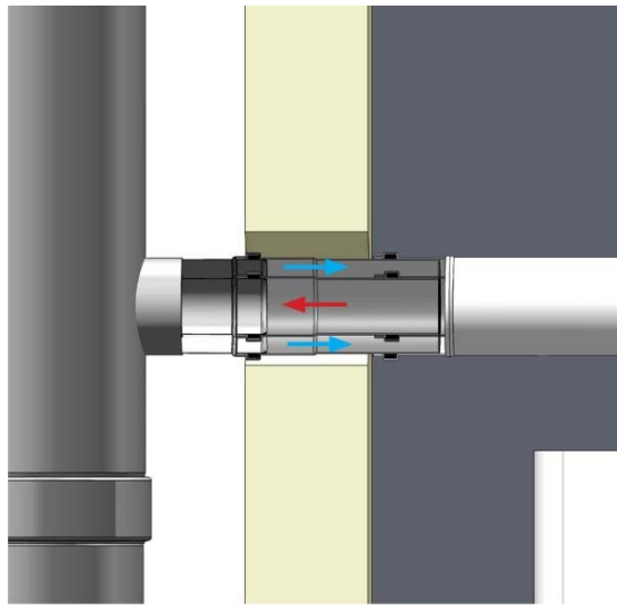
Figure 11 – Mise en place des conduits de liaison, version DINAGAS 3CE+, à l'intérieur d'un bâtiment.
