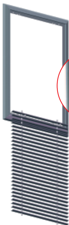
Noyau d'ailettes soutenu grâce au clip 007.
