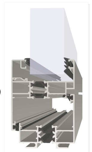
Ouverture intérieure
